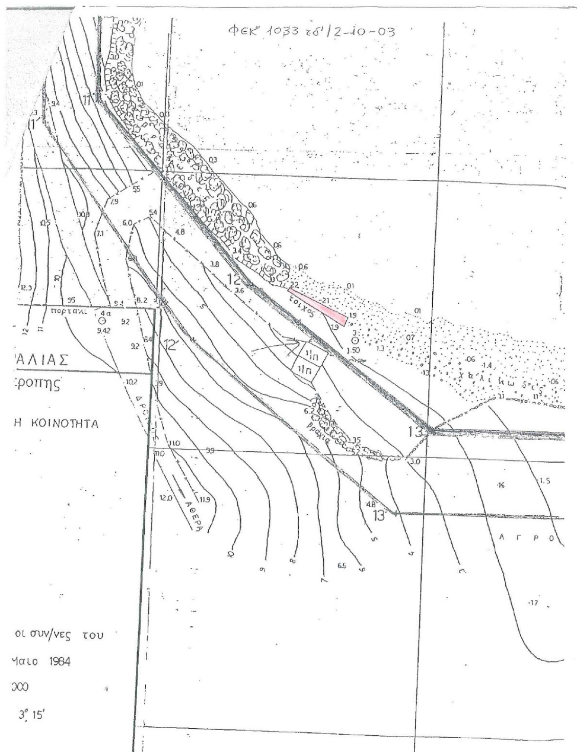
Εικόνα 6: Σκαρίφημα που περιλαμβάνεται στο υπ' αρ. πρωτ. 317/09-02-2006 Πρωτόκολλο Κατεδάφισης.
